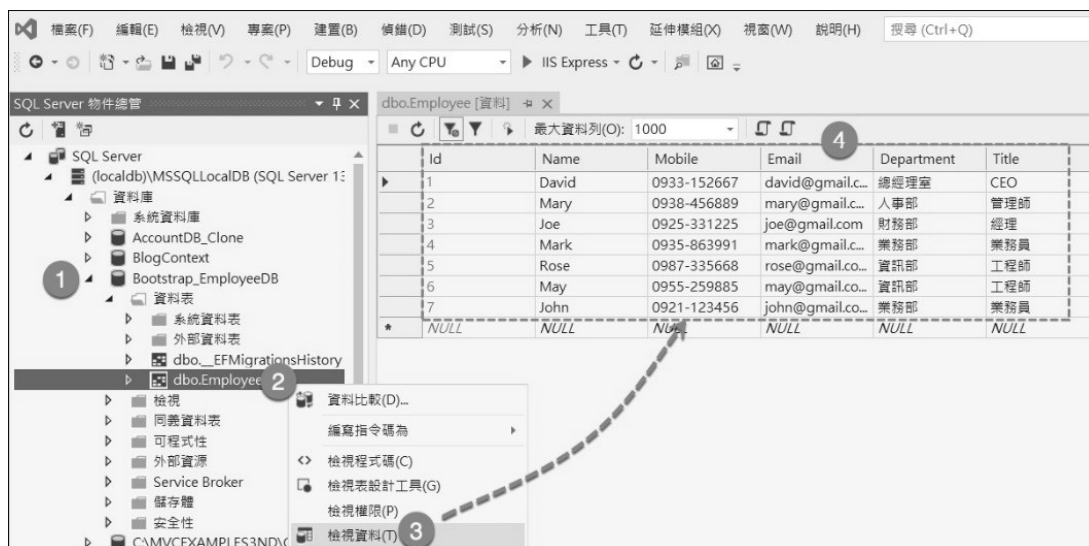
圖 6-30 用 SQL Server 物件總管察看資料庫
