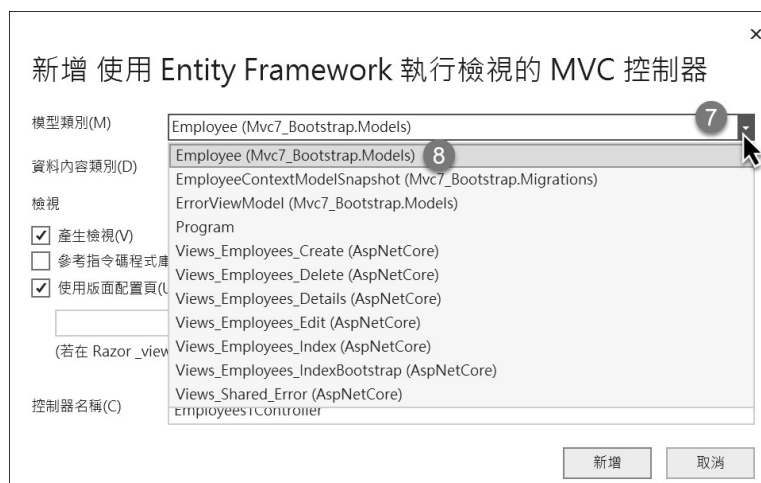
圖 6-26 指定 Employee 模型類別
