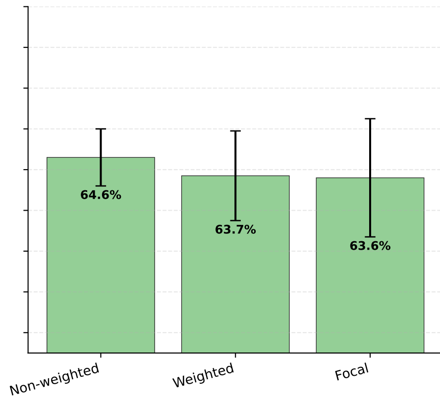
STGCN++
