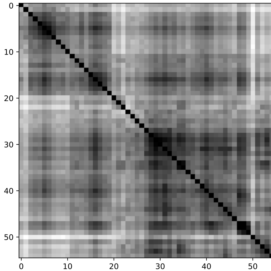
Procrustes
