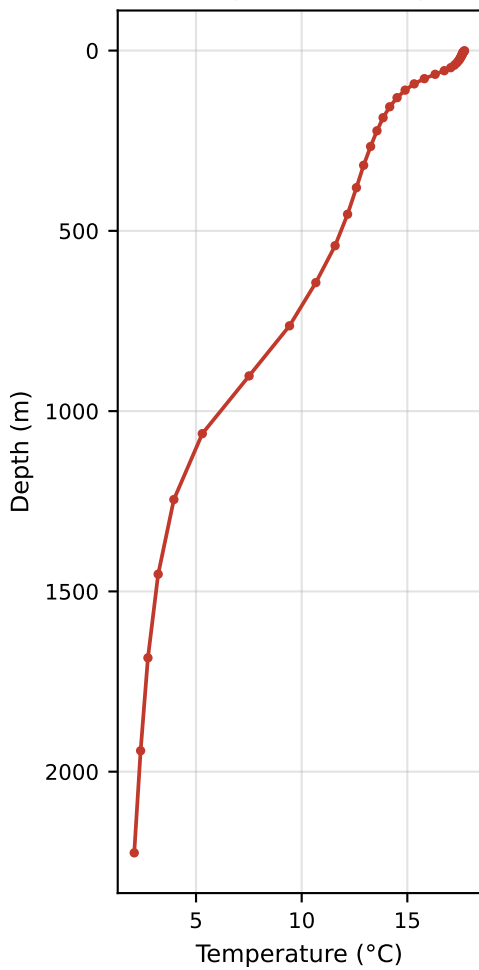
Mean Temperature (°C) profile
