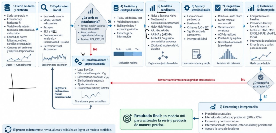
Figura 2: Flujo general para el estudio de series temporales.
