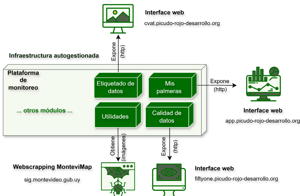
FIGURA 3.2. Diagrama de interfaces externas con sus protocolos de comunicación.
