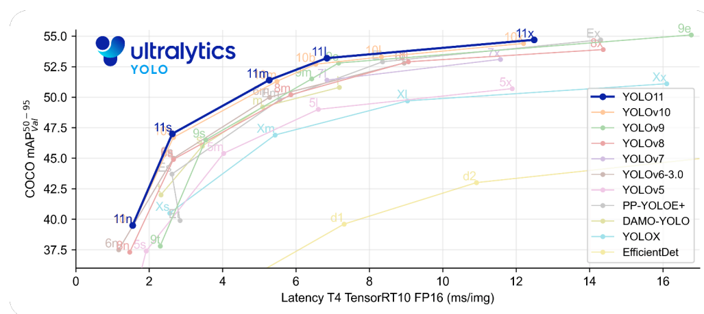
FIGURA 4.1. Comparación de performance entre YoloV11 y versiones anteriores, donde se destaca principalmente en el tiempo de inferencia, manteniendo un excelente mAP50-95 en el dataset de COCO 1 .
