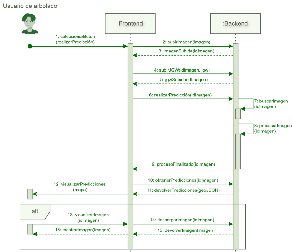
FIGURA 3.11. Diagrama de secuencia de la aplicación web Mis palmeras, mostrando el flujo de datos entre el backend y frontend.
