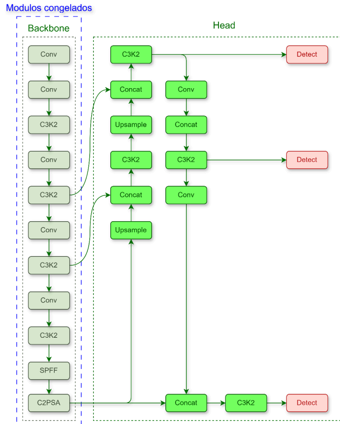
FIGURA 4.2. Esquema del enfoque de entrenamiento basado en transfer learning , en donde se especifica el congelamiento del backbone para el entrenamiento del modelo de detección del picudo rojo.
