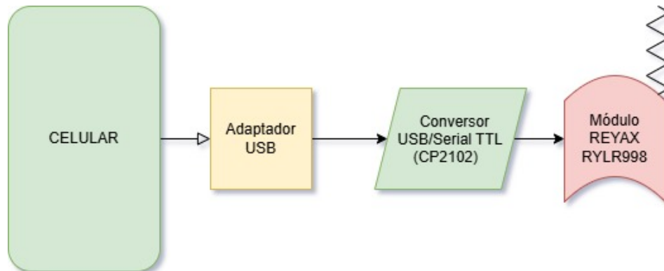
Figura 3 – Diagramas de blocos mostrando a interação do aparelho de celular com o módulo RYLR998
