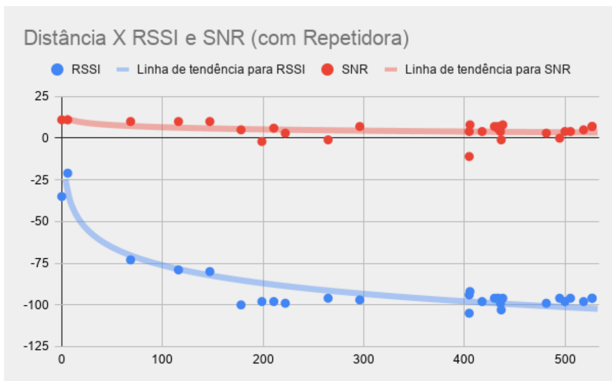
Figura 14 – Gráfico mostrando o comportamento da qualidade do sinal e relação sinal ruído considerando a distância, utilizando a Estação Repetidora. Neste caso os dados de RSSI e SNR referem-se ao último trecho, após a repetidora.
