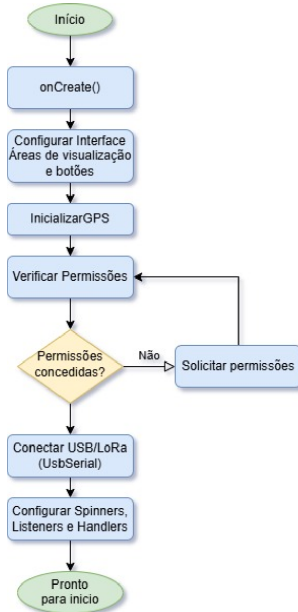
Figura 8 – Fluxograma de Inicialização do Lora SOS
