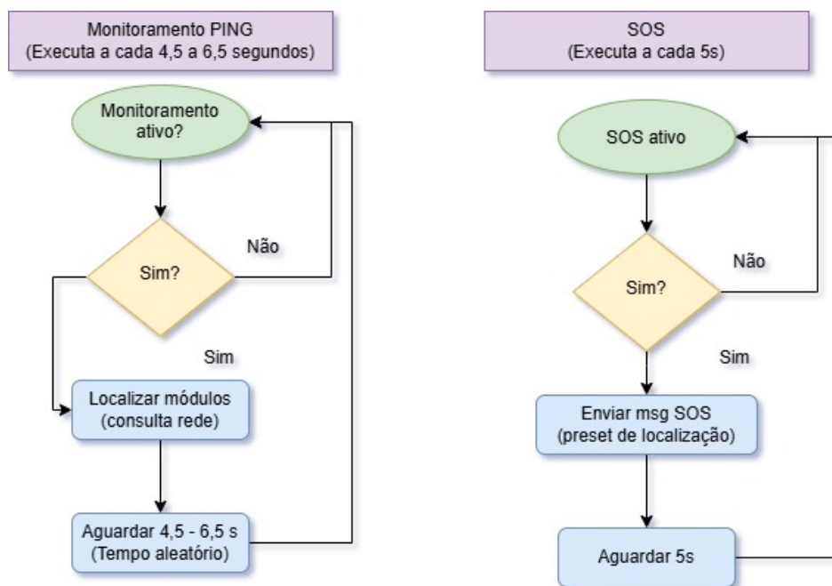
Figura 10 – Fluxo de Monitoramento / Fluxo da mensagem de SOS
