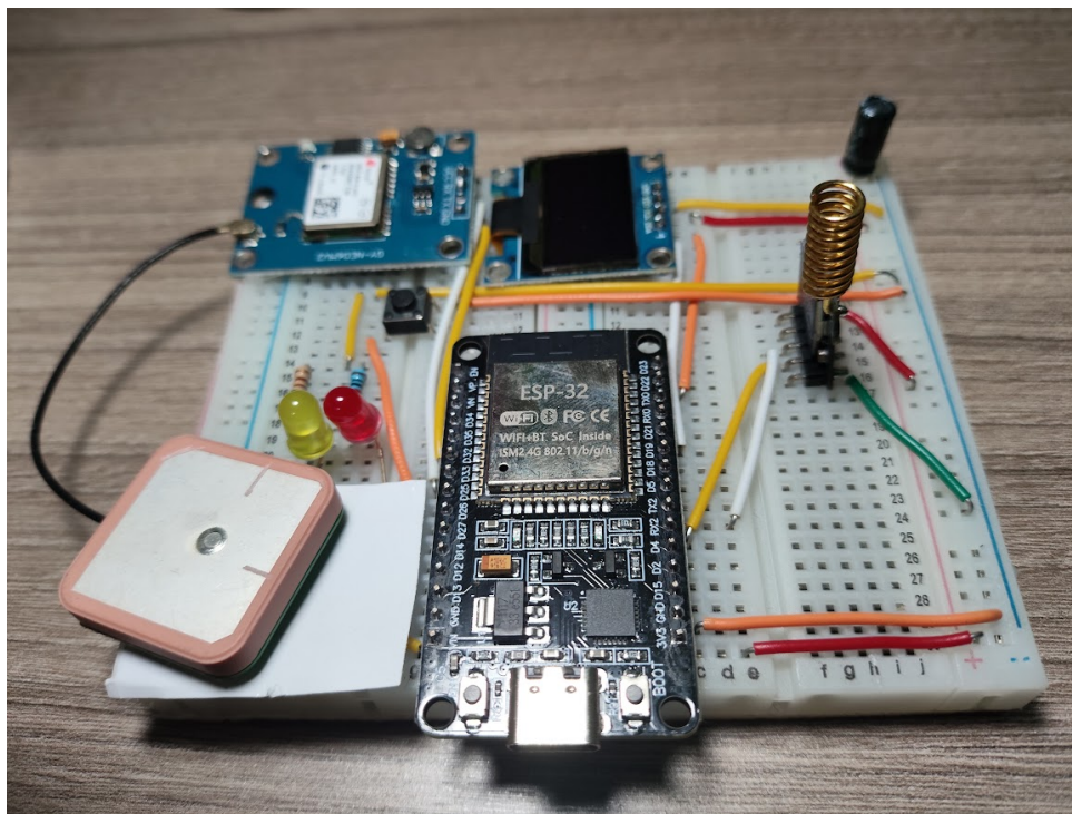
Figura 6 – Módulo Repetidor (com botão de SOS), incluindo display OLED, módulo GPS e led amarelo de recepção de pacotes
