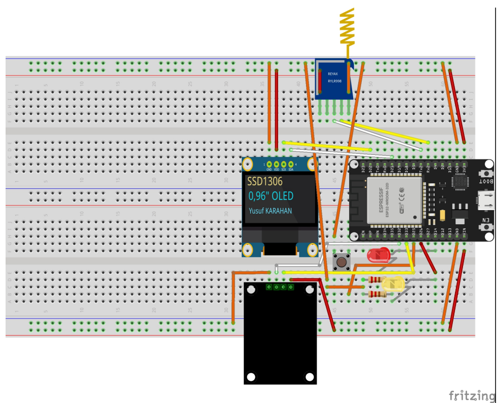
Figura 12 – Projeto visual eletrônico da Estação Repetidora utilizando o software Fritzing
