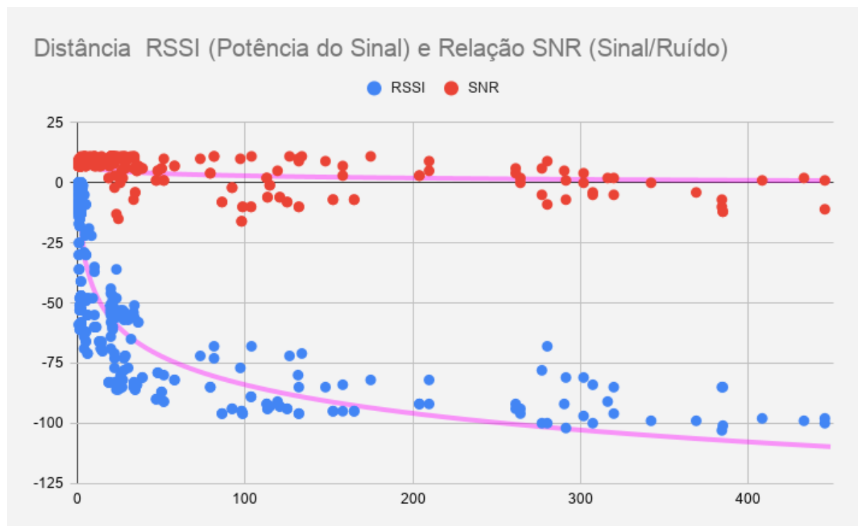
Figura 13 – Gráfico mostrando o comportamento da qualidade do sinal e relação sinal ruído em relação à distância
