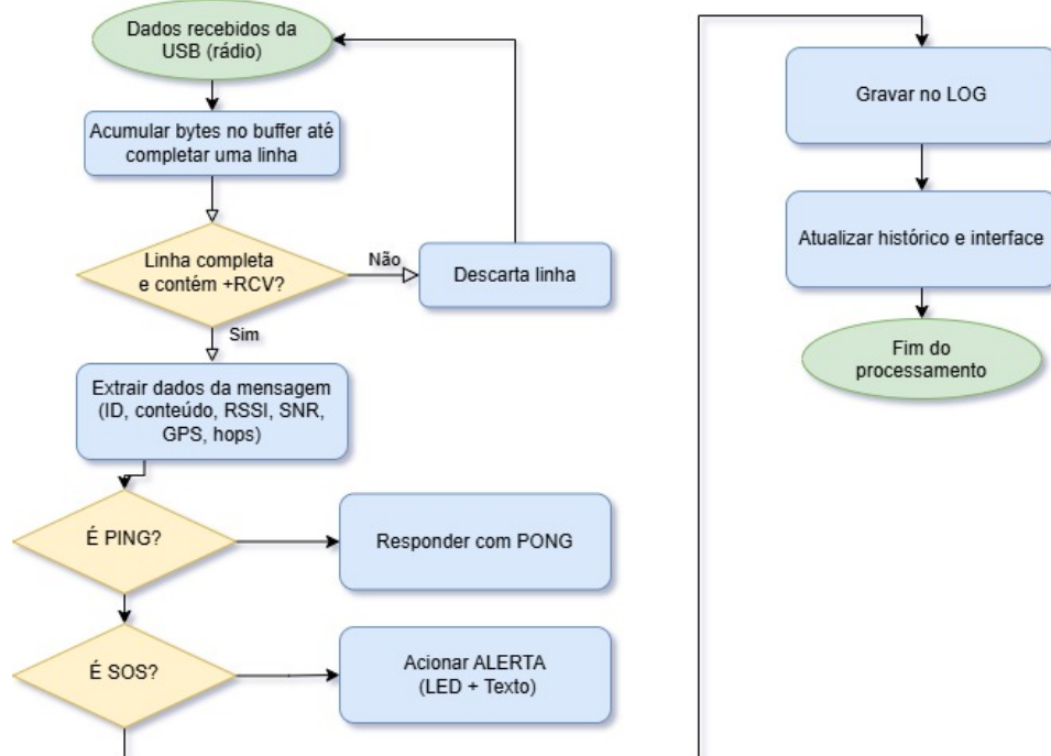
Figura 9 – Fluxo de Recepção / Processamento do App Lora SOS
