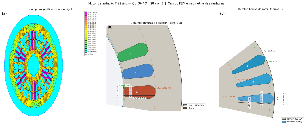
Figura 1. (a) Mapa de densidade de campo |B| (Config. I, normalizado B_{g,1}=0,9 T). (b) Detalhe das ranhuras do estator (slots 1–3) com cotas principais. (c) Detalhe das barras do rotor (barras 1–3) com cotas principais.
