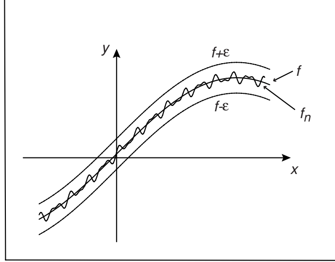
FIGURA 5.2. Convergencia uniforme
