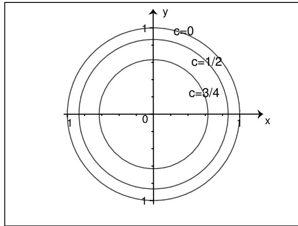
FIGURA 12.4. curvas de nivel de f(x, y) = \sqrt{1 - x^2 - y^2}
