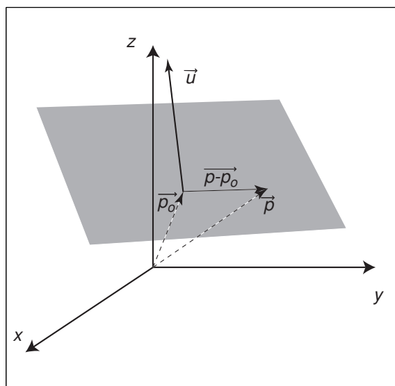
FIGURA 7.8. Plano que pasa por \vec{p}_o y es perpendicular a \vec{u}
