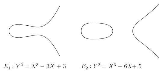
Fig. 1.2: Dos ejemplos de curvas elípticas en el eje cartesiano de los reales
