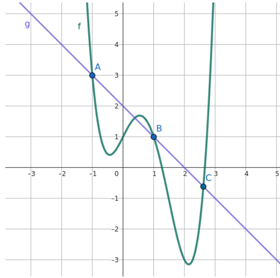
Fig. 1.1: Intuición de intersección de polinomios en R^2
