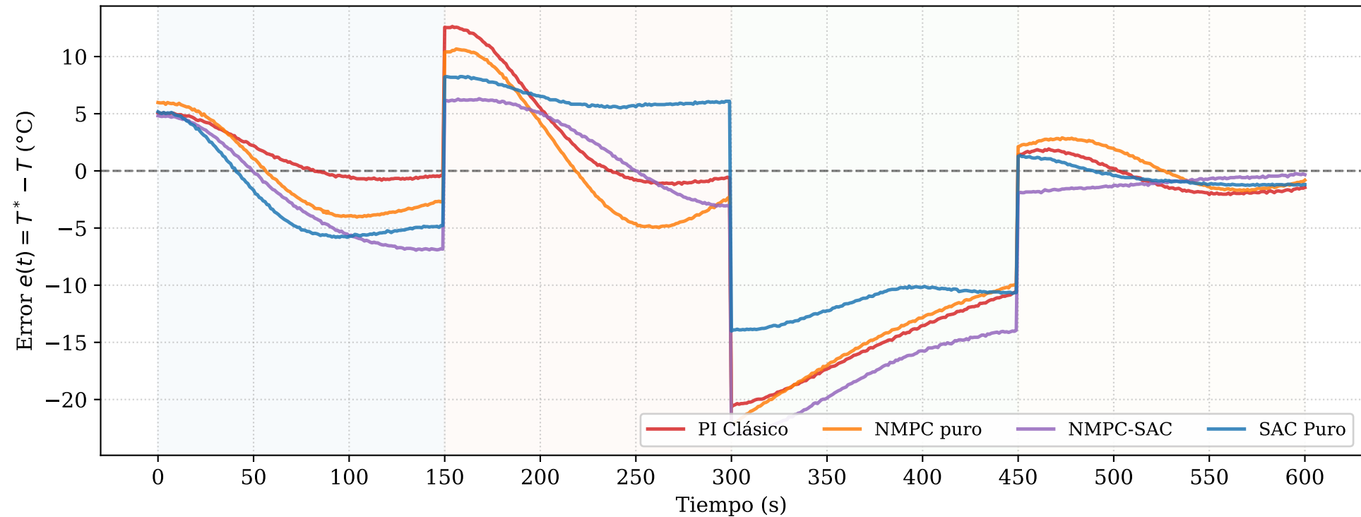
Trayectoria del Error de Seguimiento — 4 Controladores
