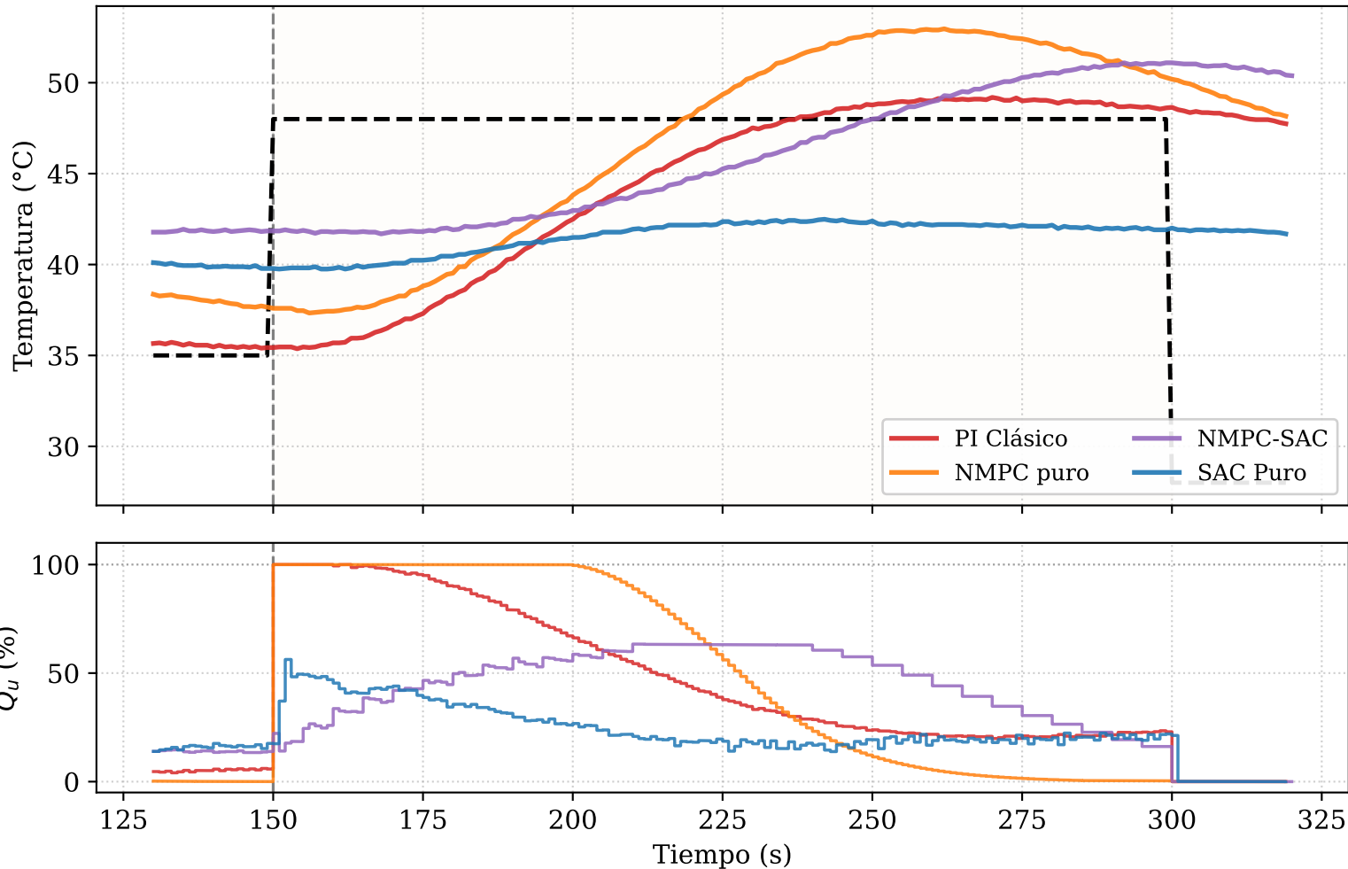
Zoom: Escalón de Calentamiento +13°C ( t = 150\text{s} ) — Windup y Anticipación
