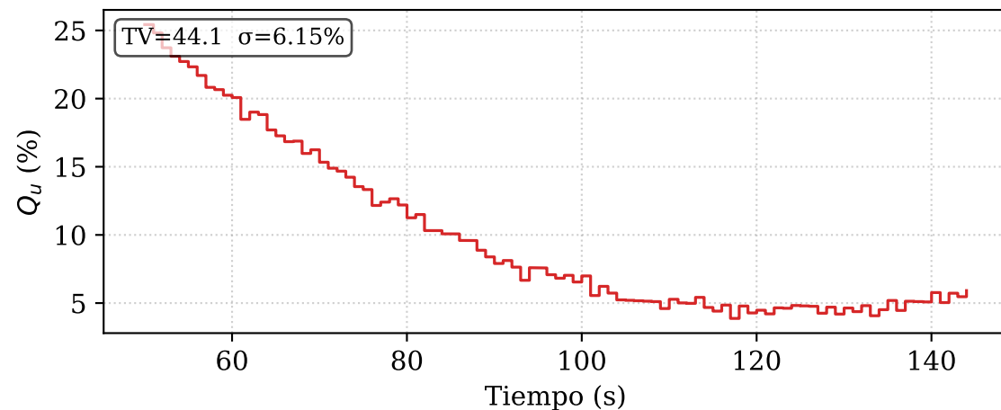
Señal Q_u(t) — PI Clásico
