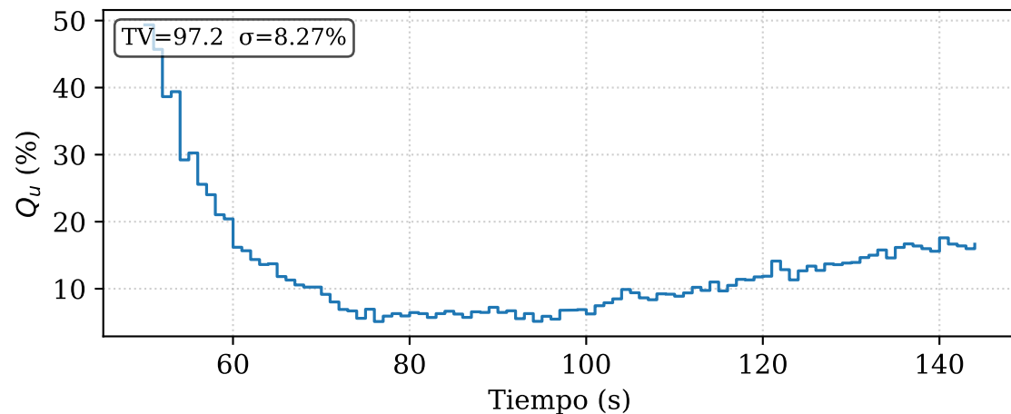
Señal Q_u(t) — SAC Puro
