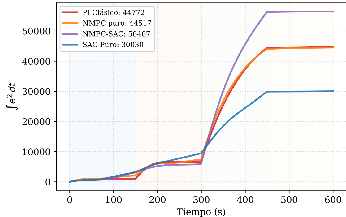
ISE Acumulado
