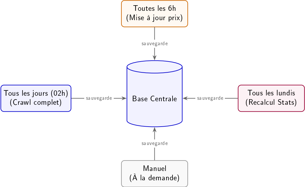
Diagramme S8 — Le Cycle Automatique
