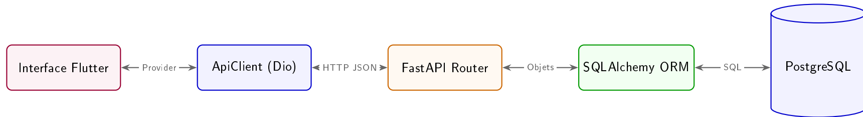
Diagramme 10 — Flux de Requêtes API
