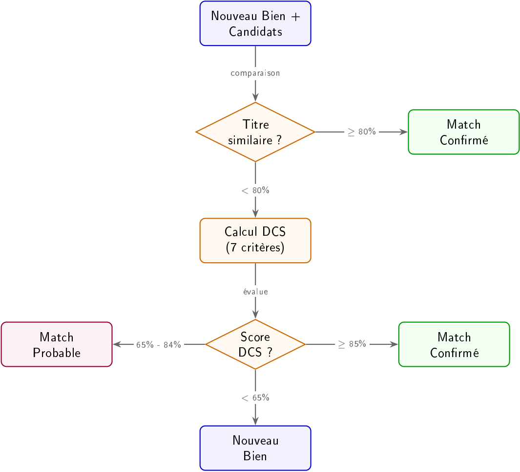
Diagramme 7 — Résolution des Doublons (DCS)
