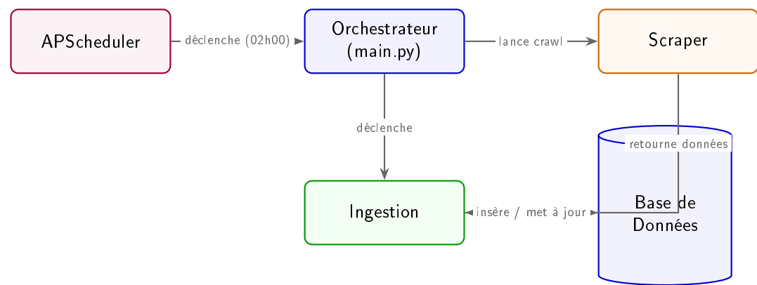
Diagramme 6 — Orchestration des Crawls
