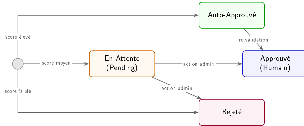
Diagramme 11 — Machine à États (Validation)
