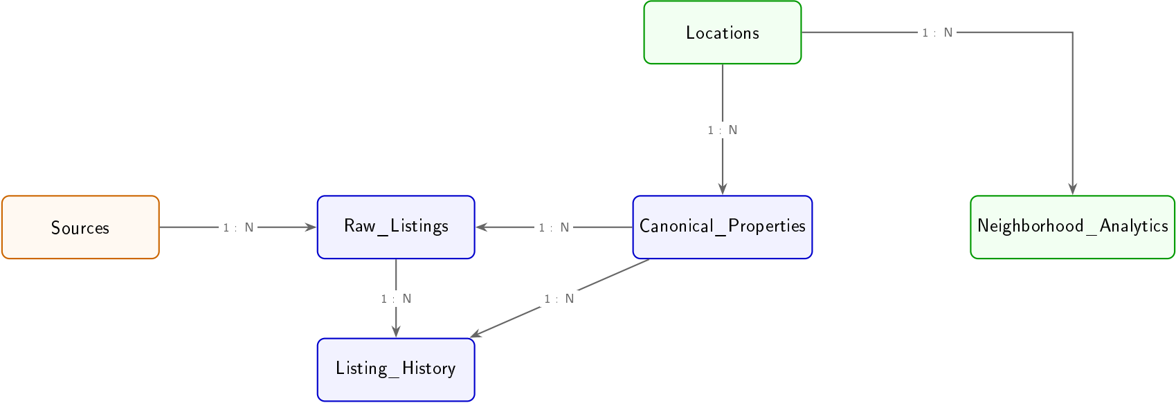
Diagramme 3 — Modèle de Données (Relations Clés)
