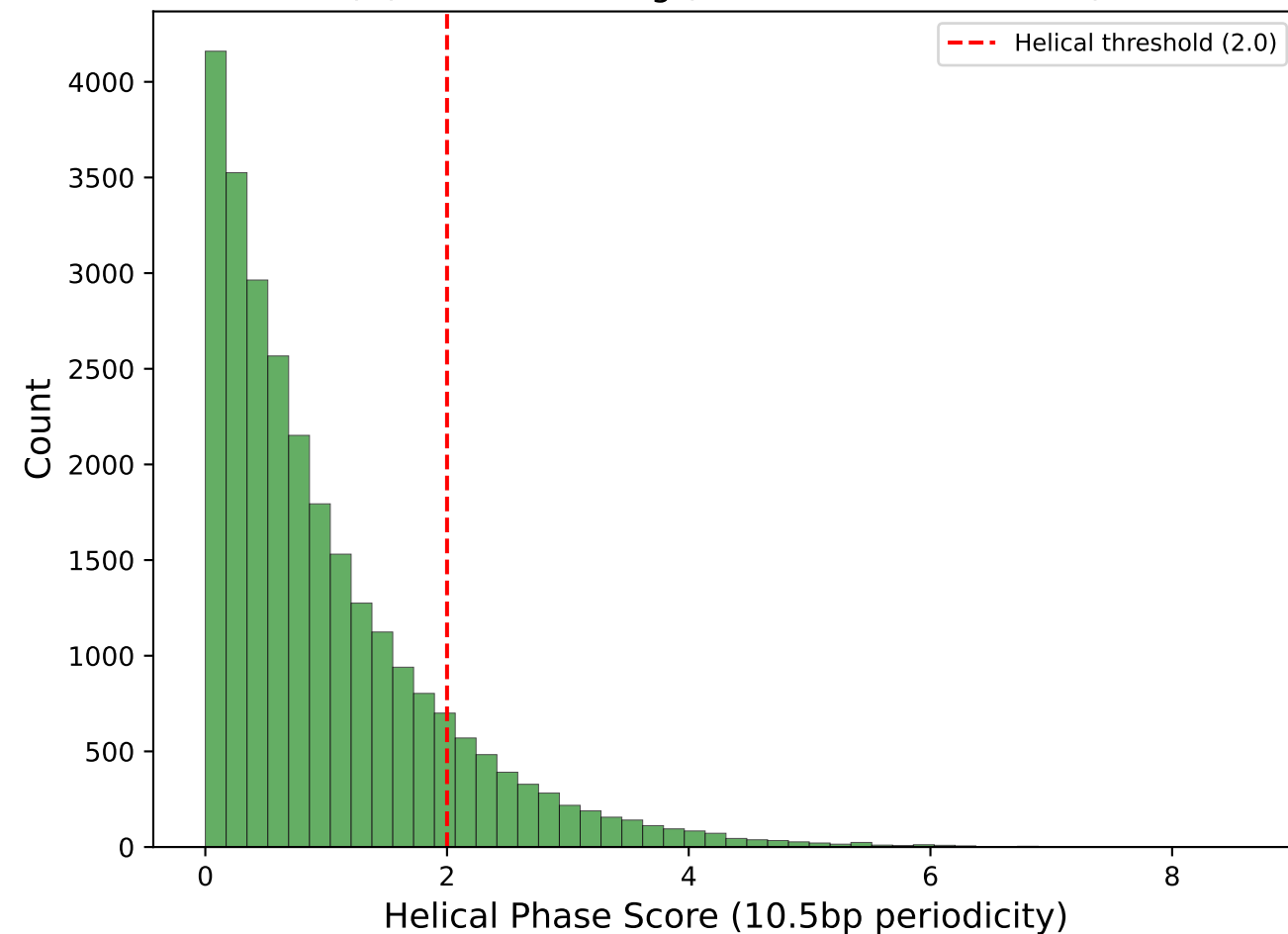
(D) Helical Phasing (3632 rules > threshold)
