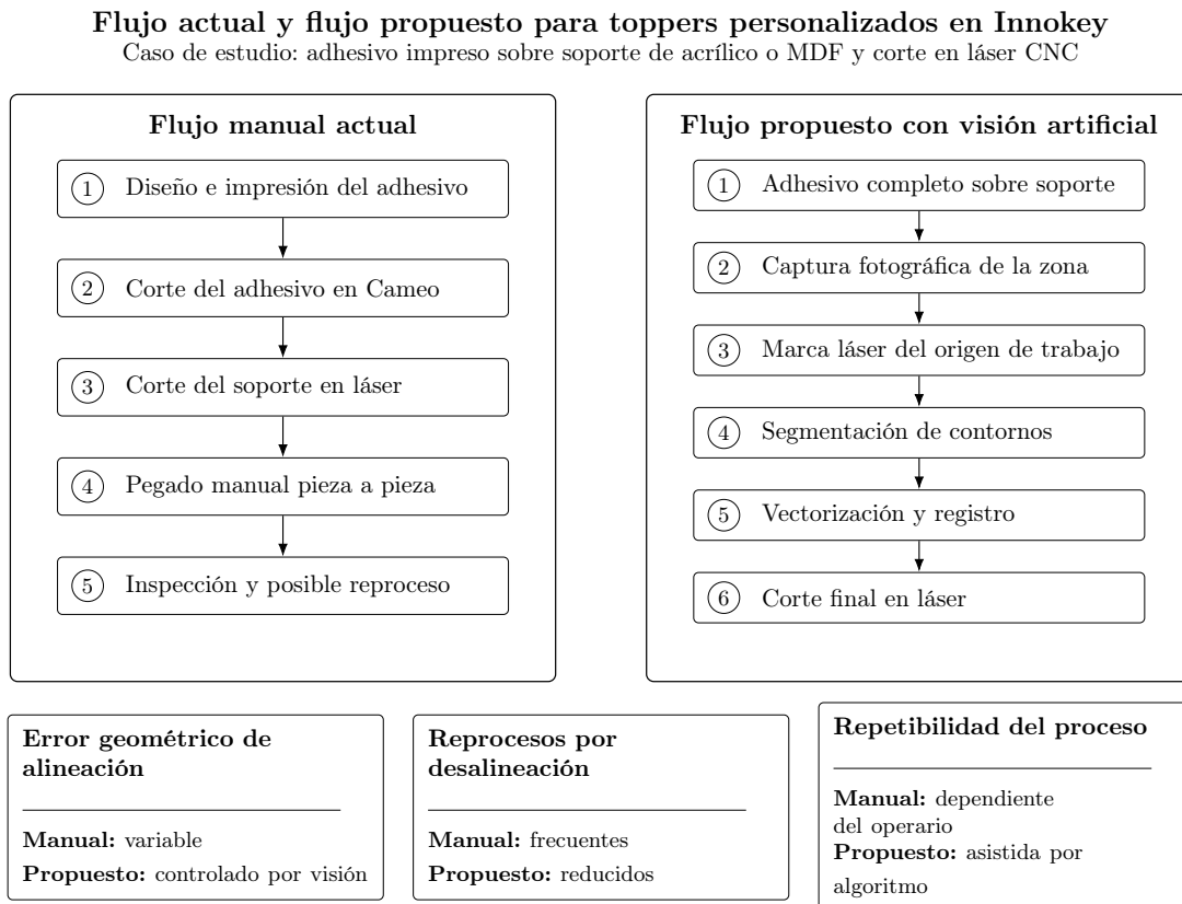
Figura 1.1: Comparación entre el flujo manual actual y el flujo propuesto para la fabricación de toppers en Innokey.
