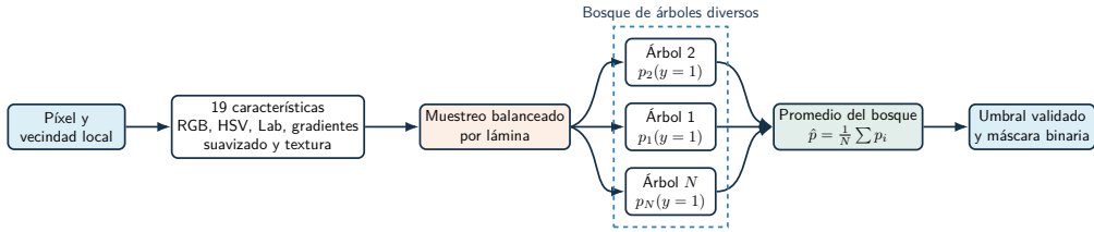
Figura 2.3: Funcionamiento del Random Forest por píxel, desde la extracción de características hasta la agregación de los árboles y la formación de la máscara.
