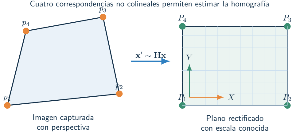
Figura 2.2: Rectificación de la hoja mediante correspondencias entre los marcadores detectados y el plano canónico A4.
