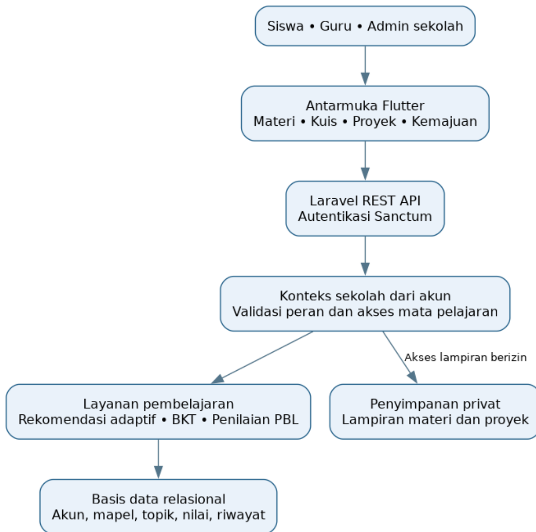
Gambar C.1. Arsitektur ringkas Flutter-Laravel. Permintaan data melewati autentikasi, konteks sekolah, dan pemeriksaan akses. Diagram menampilkan jalur utama, bukan seluruh komponen deployment.
