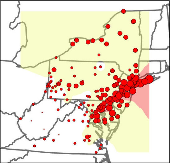
Kriging
