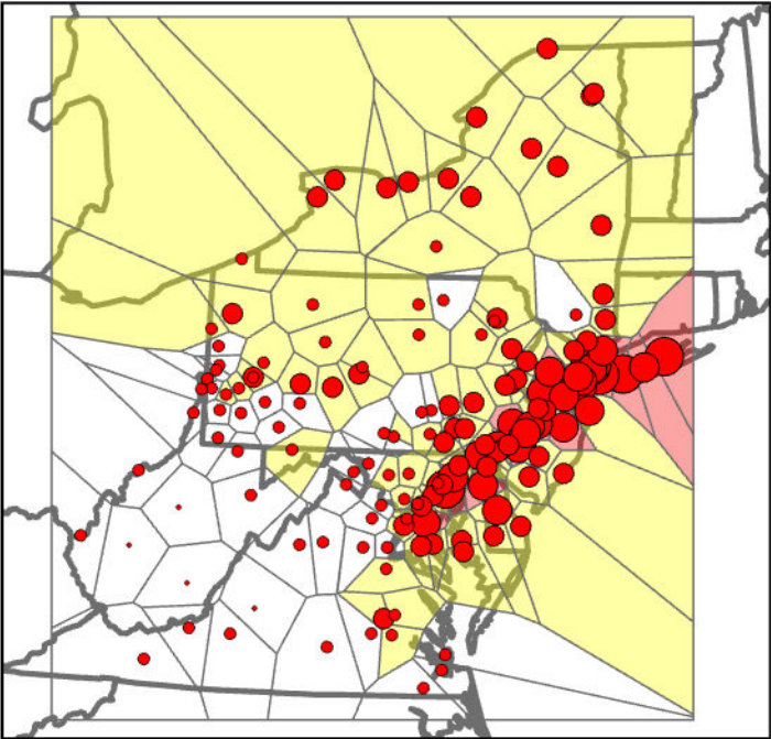
Kernel
