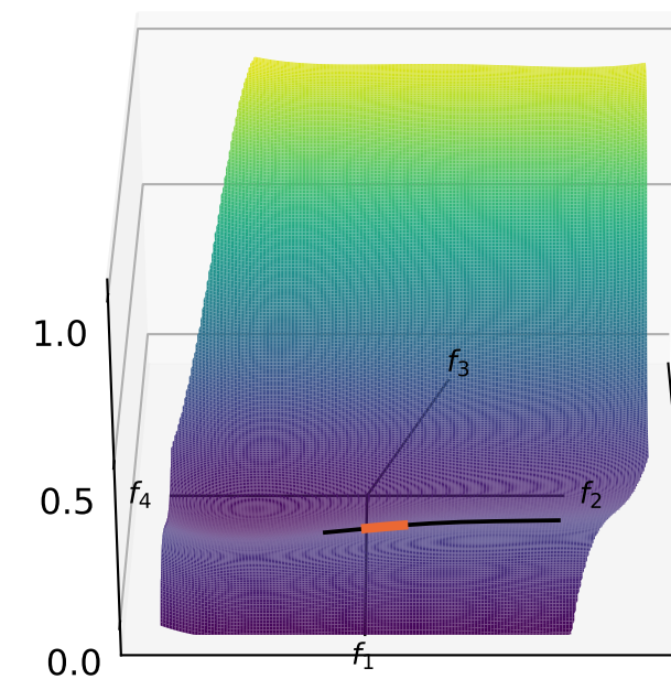
tied ReLU
