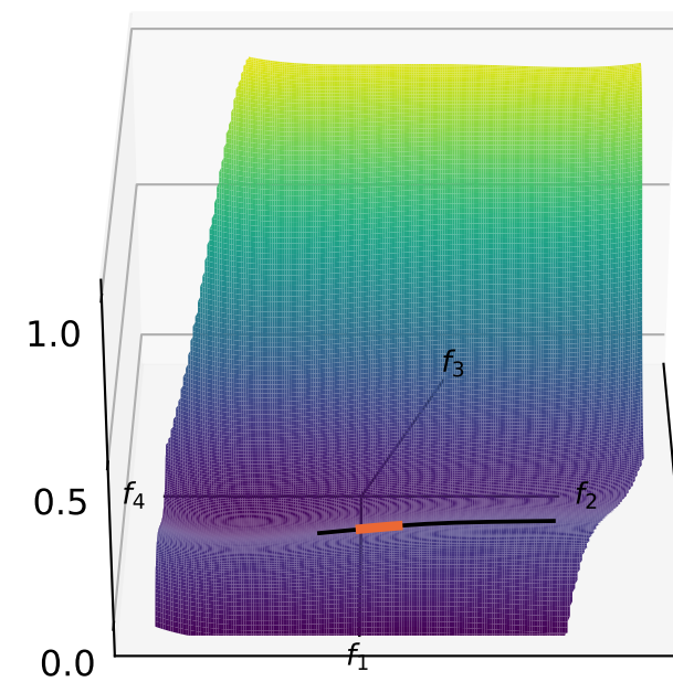
tied ReLU
