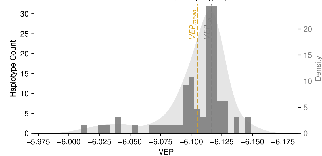
SMARCAL1:D816E (74 haplotypes)
