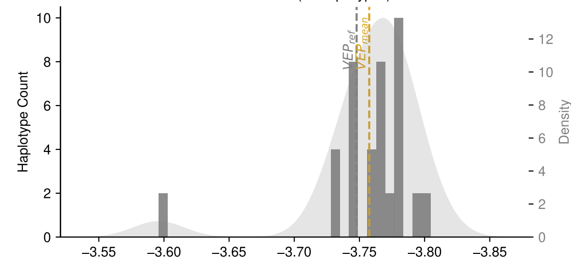
SMARCAL1:D816E (74 haplotypes)
