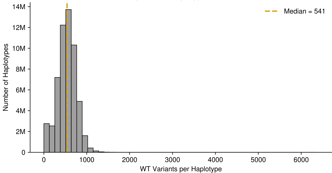
WT Variants per DNA Haplotype (524 kb windows)
