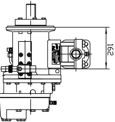
Rückwärtige Ansicht Rear View
