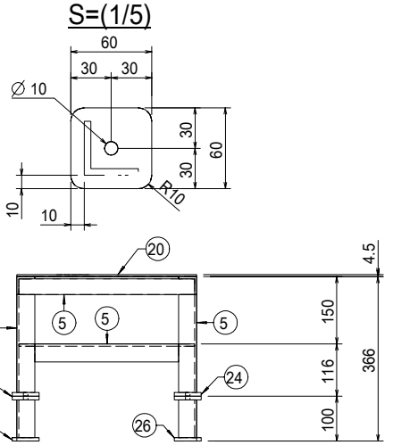
DET. ㉔ (4EA)
