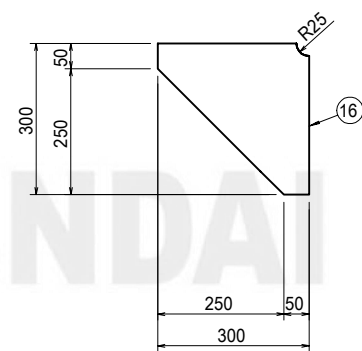
DET. 'z-3A' (1EA) (S=1:15)
