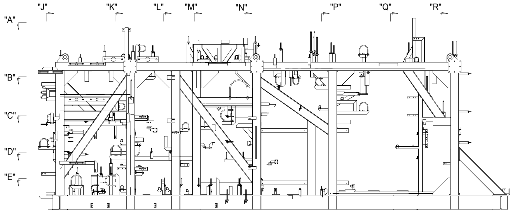
KEY ELEVATION
