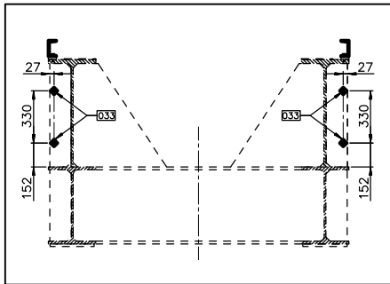
SECTION D-D
