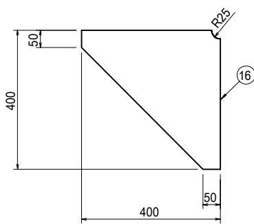
DET. 'z-3' (20EA) (S=1:15)
