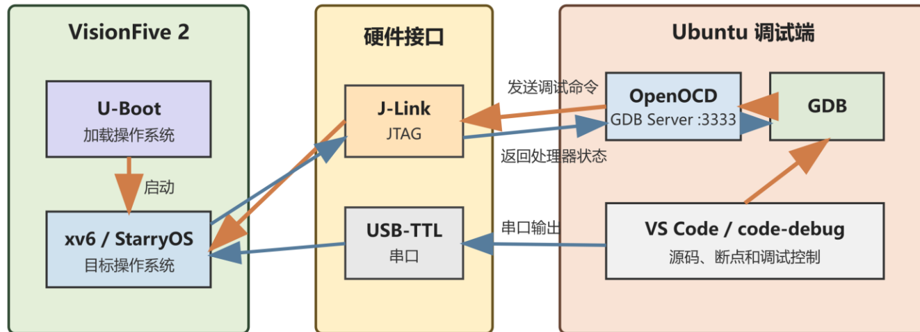
硬件调试通信示意图
