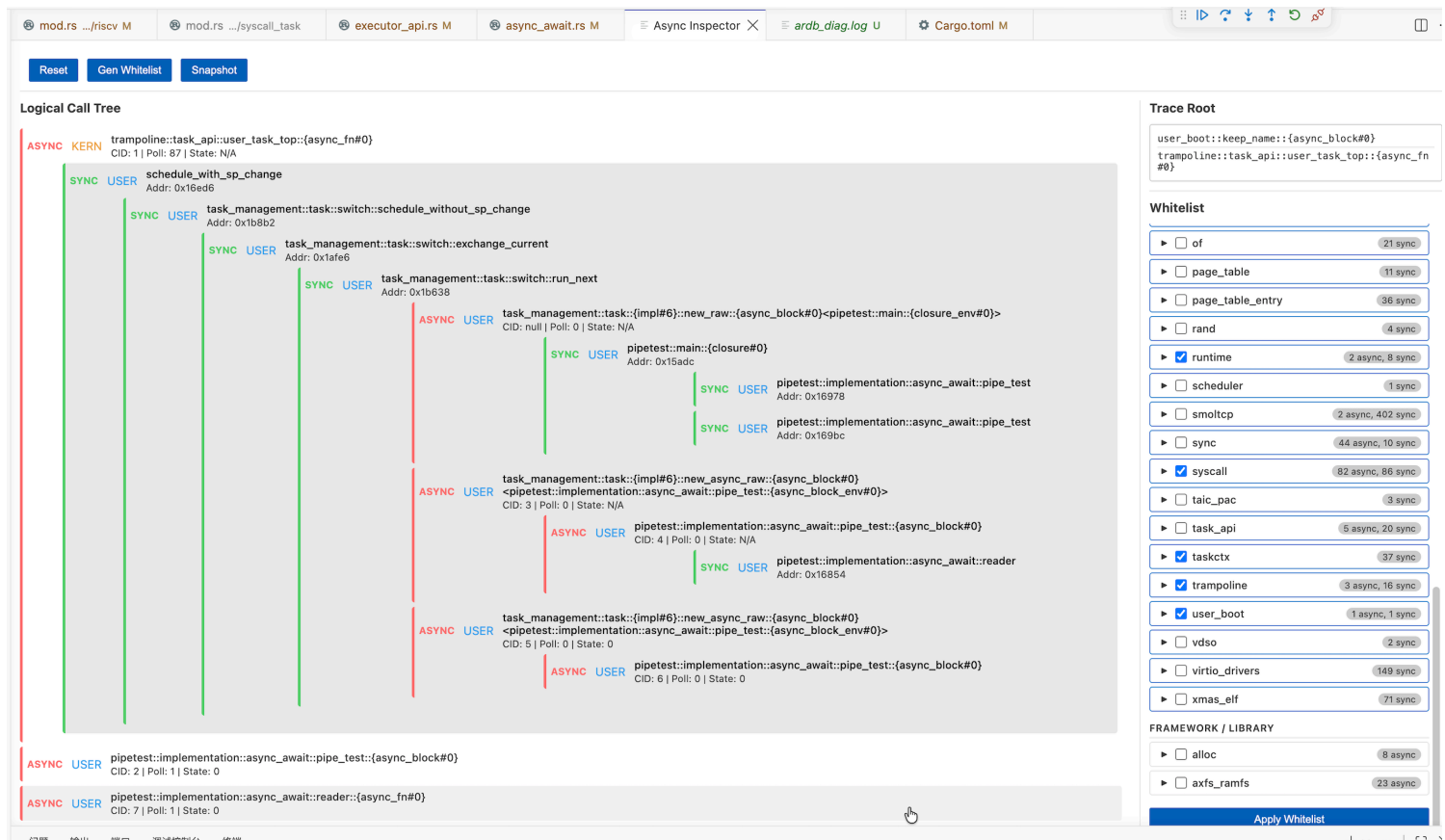
图 5: 贯穿内核态与用户态的调用树
