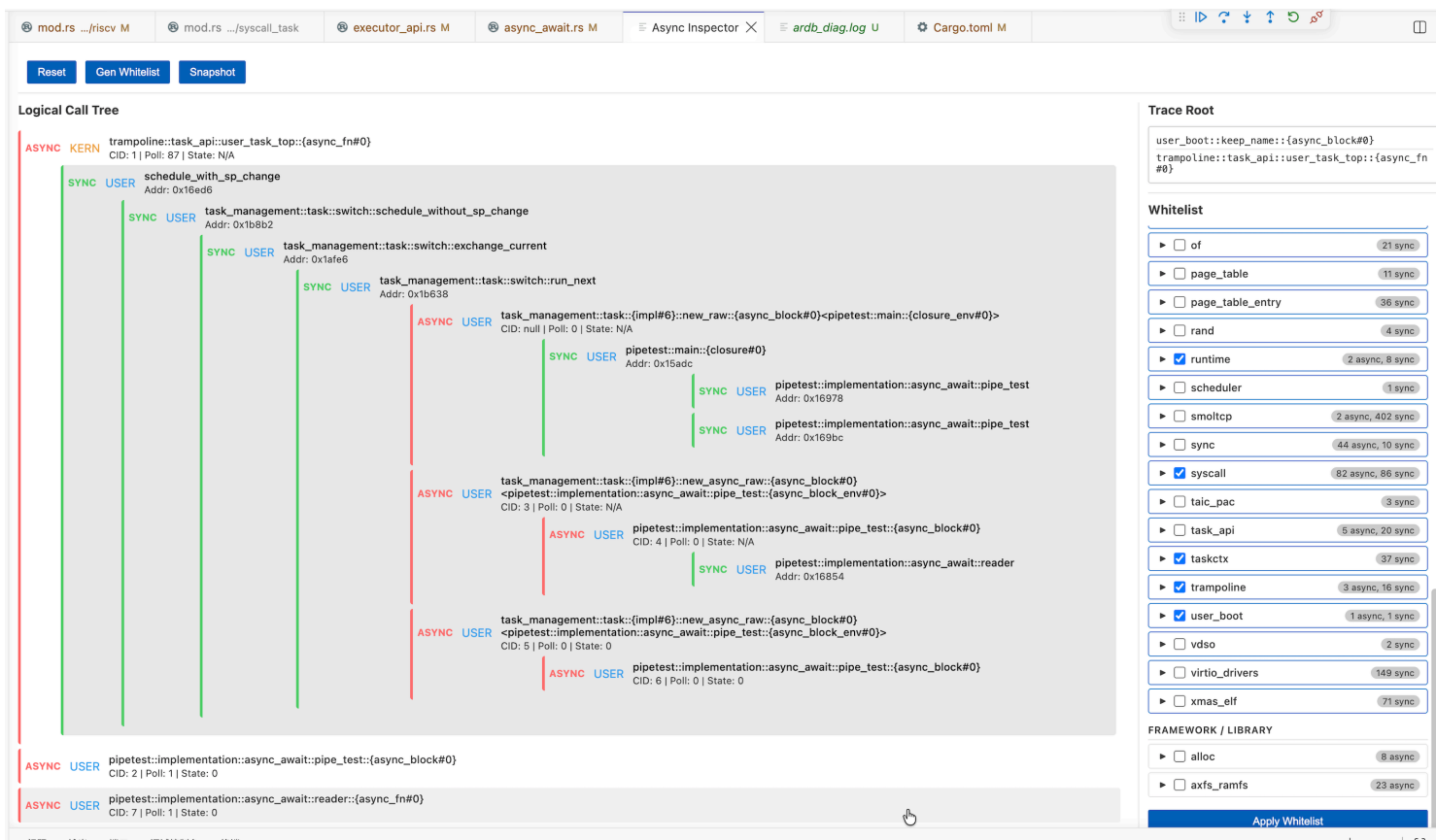
图 20: pipetest 断点 4（writer 入口）命中的调用树
