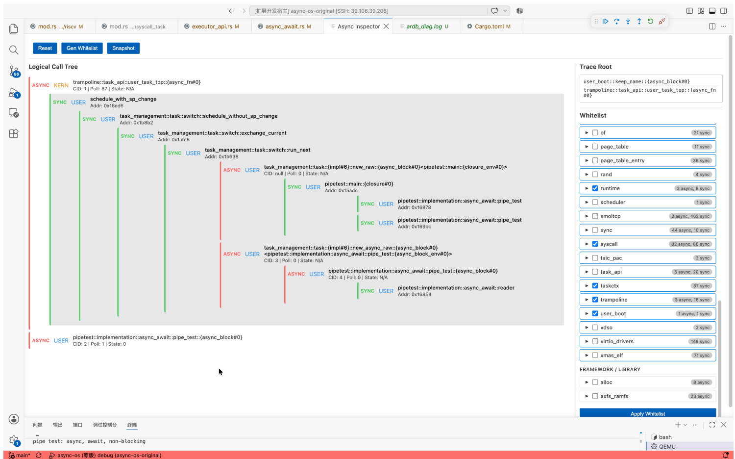
图 18: pipetest 断点 3 (reader 入口) 命中的调用树
