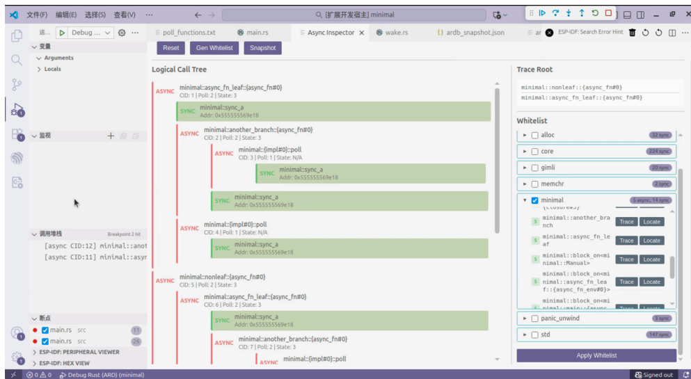
图 7: Async Inspector Webview 面板：左侧为逻辑调用树视图（红色 async 节点、绿色 sync 节点，标注 CID 和 poll 次数），右侧为按 crate 分组的白名单列表（含 Gen/Apply/Trace 按钮）
