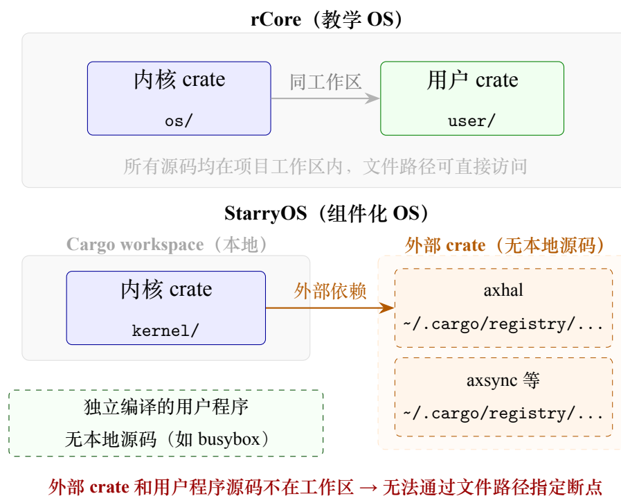
图 9: rCore 与 StarryOS 的架构差异。教学 OS 所有源码同处一个工作区，组件化 OS 的切换边界位于外部 crate，用户程序独立编译。
