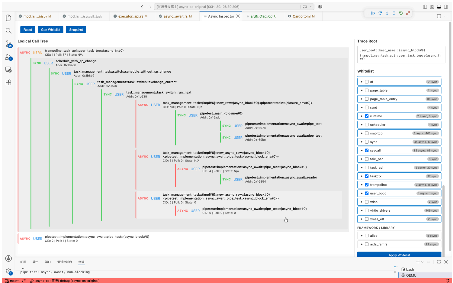
图 19: pipetest 断点 2 (spawn writer) 第 2 次命中的调用树
