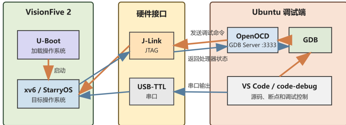
硬件调试通信示意图
