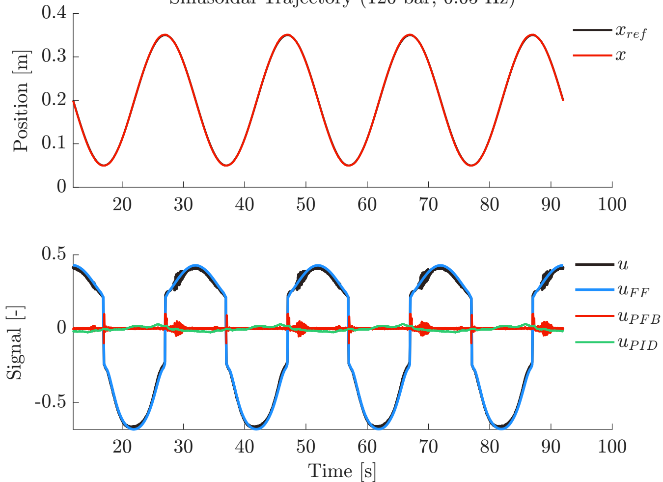
Sinusoidal Trajectory (120 bar, 0.05 Hz)
