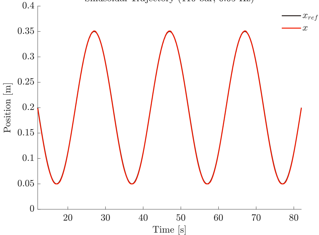
Sinusoidal Trajectory (110 bar, 0.05 Hz)
