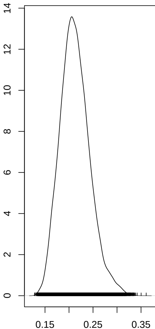
tau2.int
