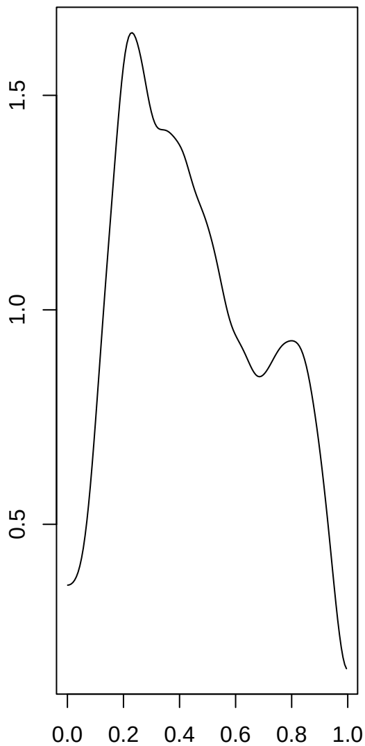
rho.slo
