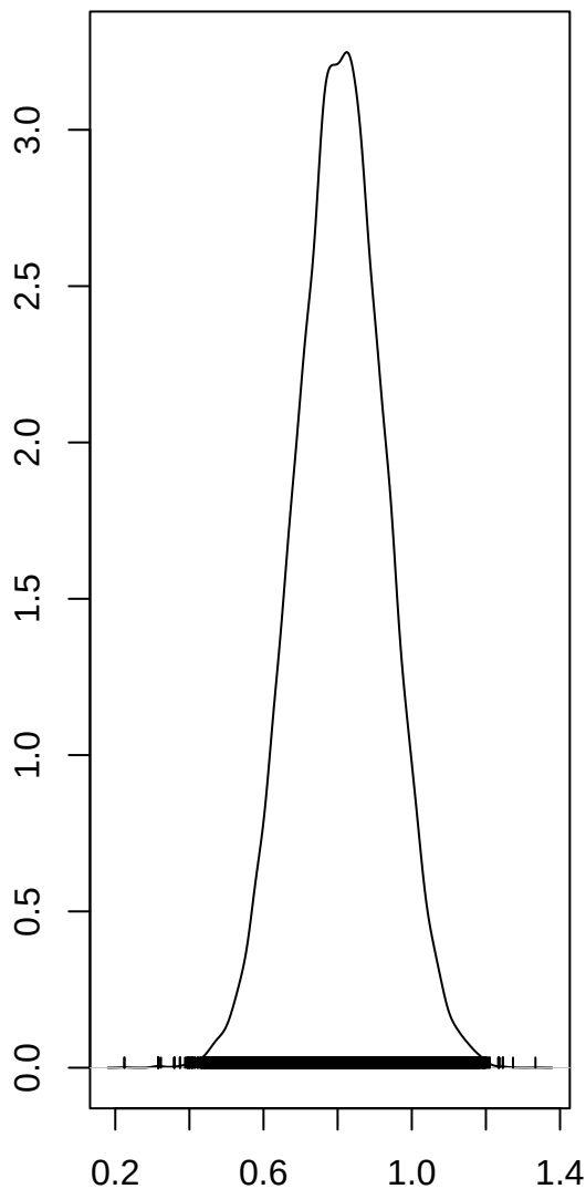
dep_rate
