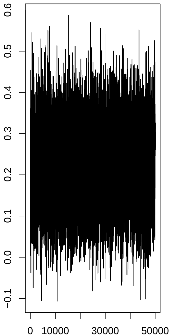
ptsd_rate
