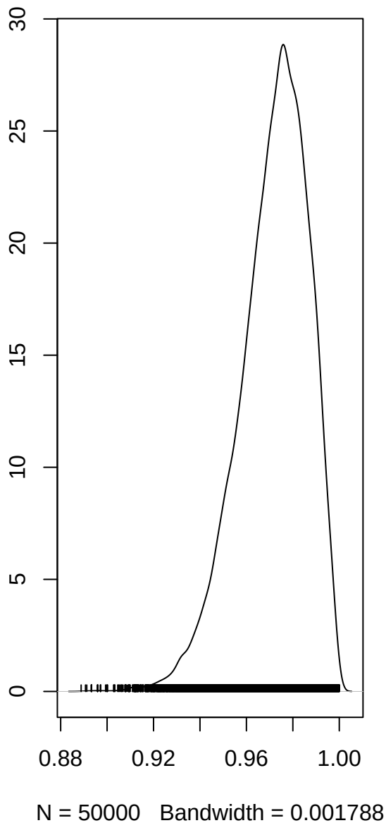
rho.int
