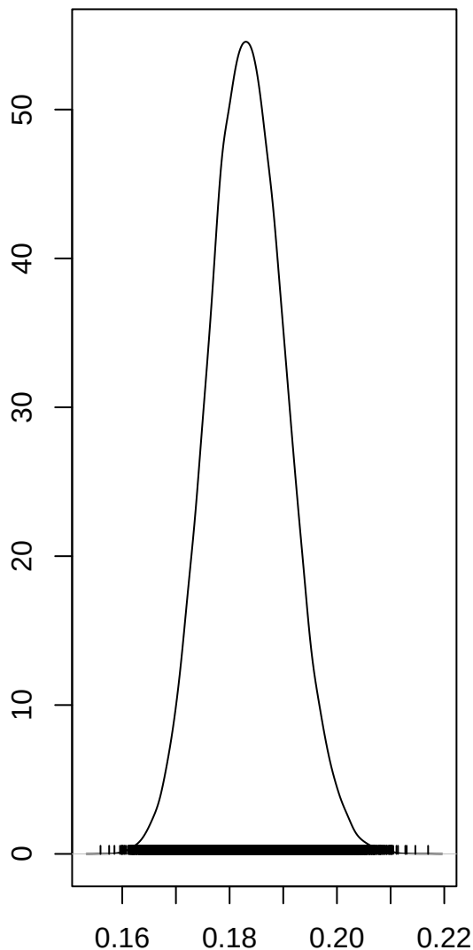
tau2.int
