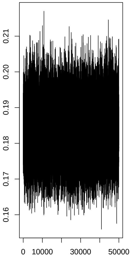
tau2.int
