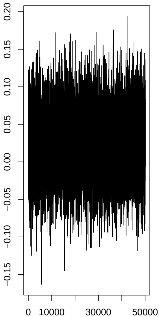
ptsd_rate
