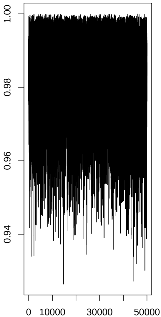
rho.int
