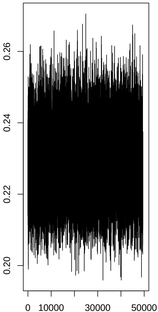
tau2.int
