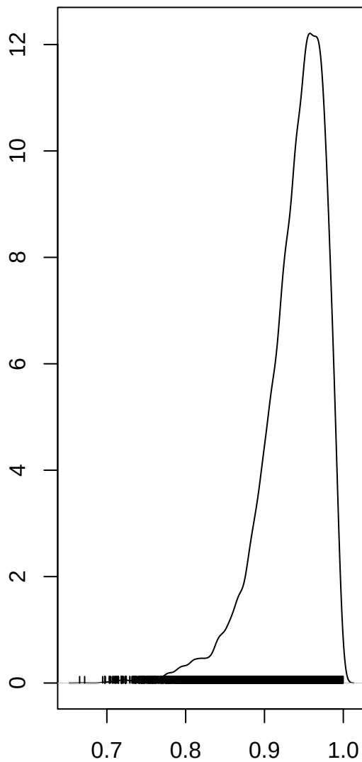
rho.slo
