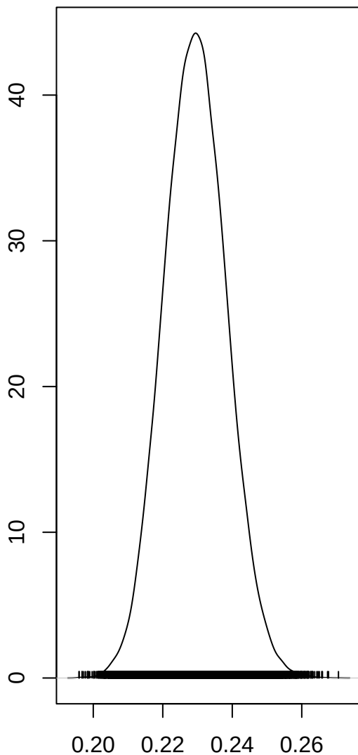
tau2.int
