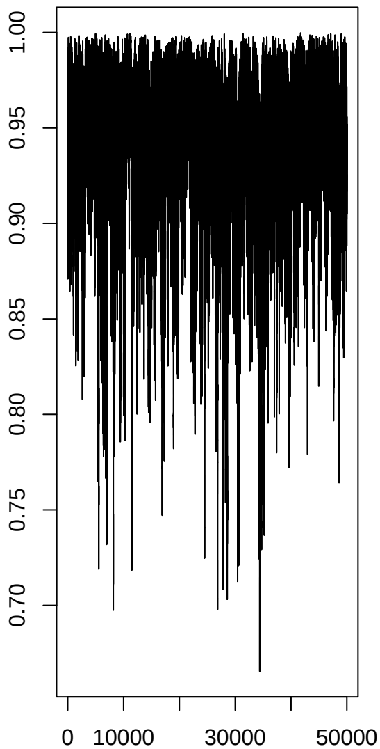
rho.slo
