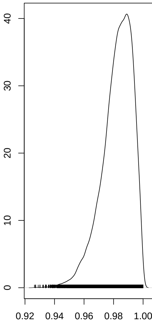
rho.int
