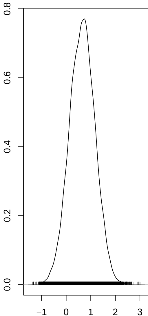
ptsd_rate
