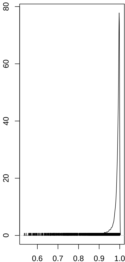
rho.int
