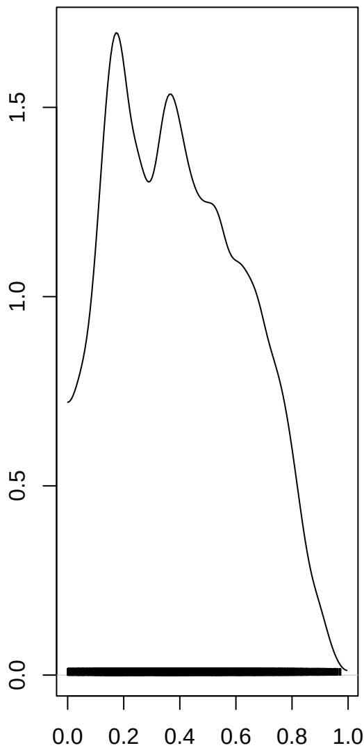
rho.slo
