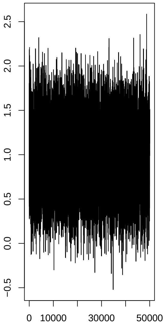
si_rate
