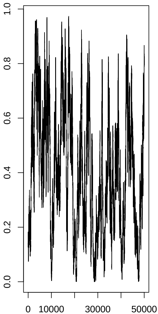
rho.slo
