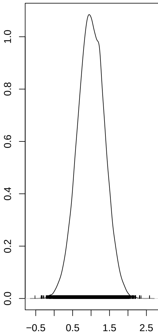
si_rate
