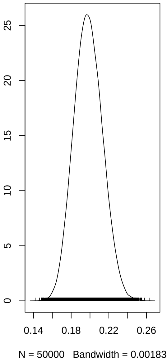
tau2.int
