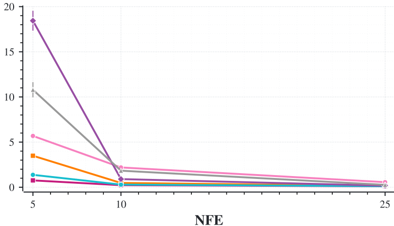
Pixel FID
