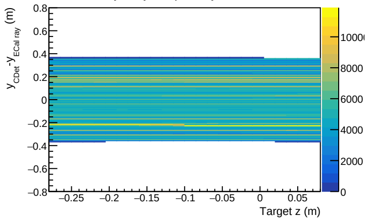
Layer 1 y compatibility residual
