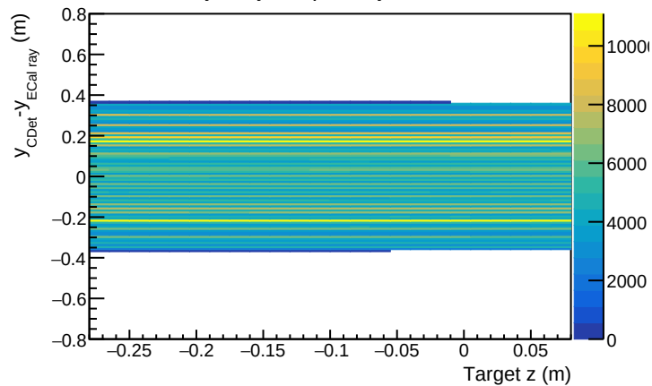
Layer 2 y compatibility residual
