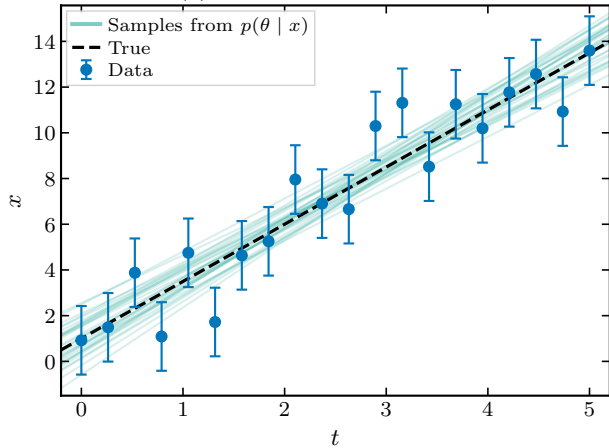
(a) Data + posterior samples
