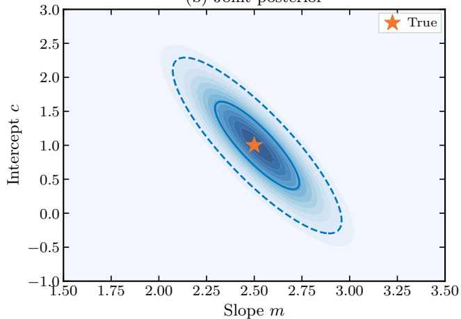
(b) Joint posterior
