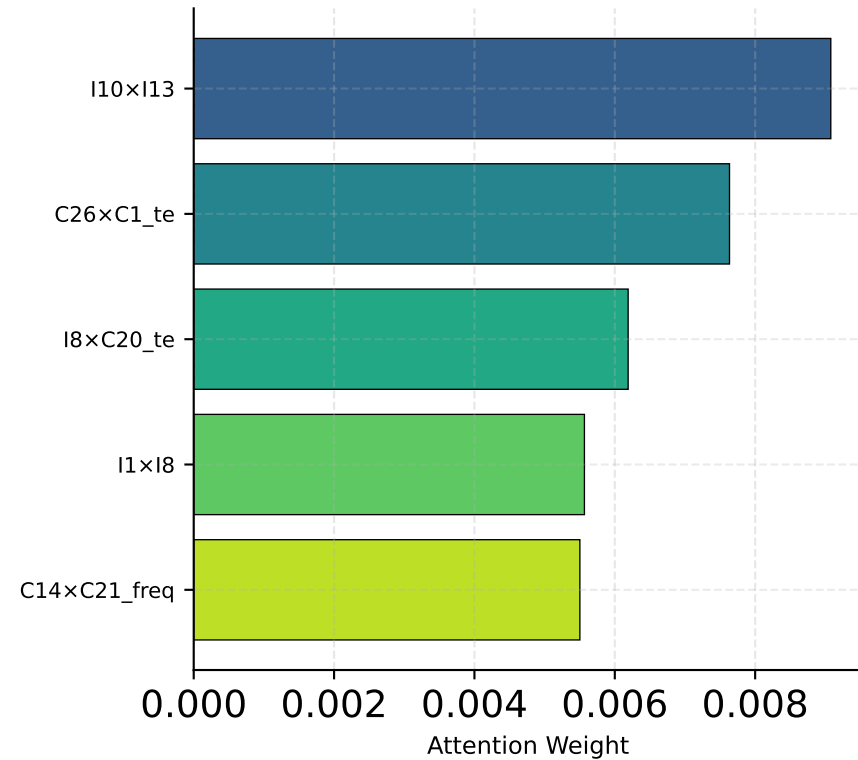
Criteo
