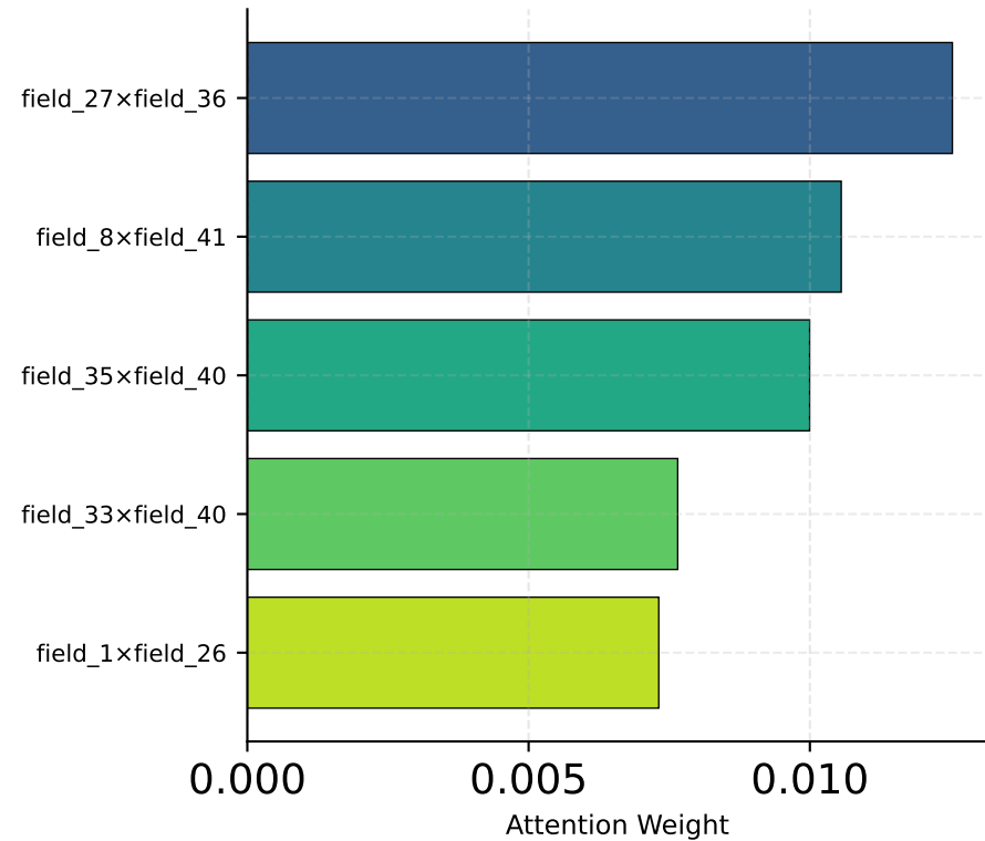
Avazu
