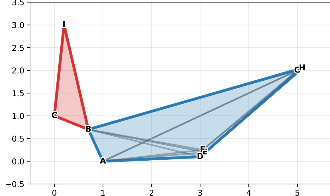
Tolerance Cliques ( \tau=0.70 ) 2 maximal cliques
