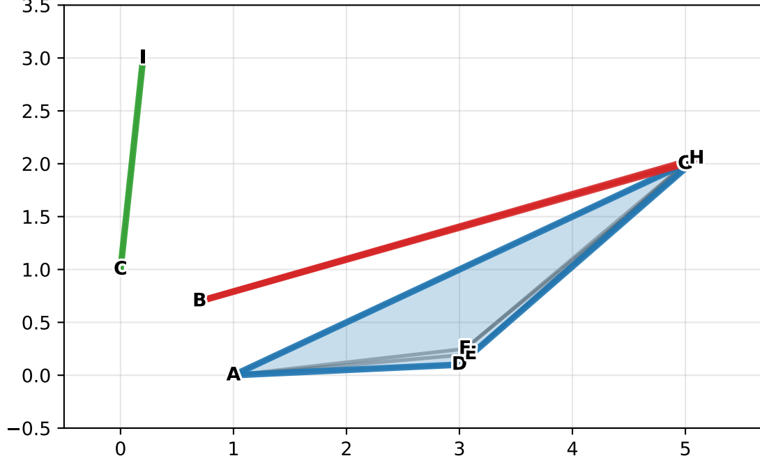
Tolerance Cliques ( \tau=0.85 ) 3 maximal cliques
