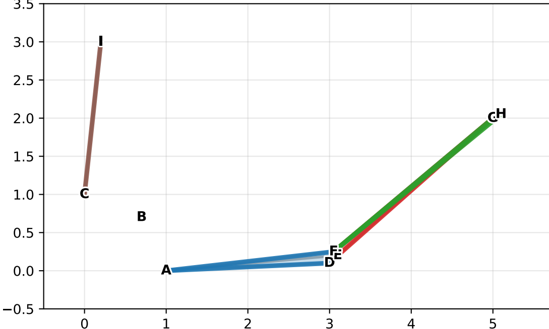
Tolerance Cliques ( \tau=0.95 ) 5 maximal cliques
